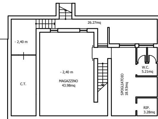
SCUOLA DELL'INFANZIA "G.SANTUCCI" "Strada Pian della Genna - MADONNA ALTA" PIANTA PIANO SEMINTERRATO - SCALA1:100
